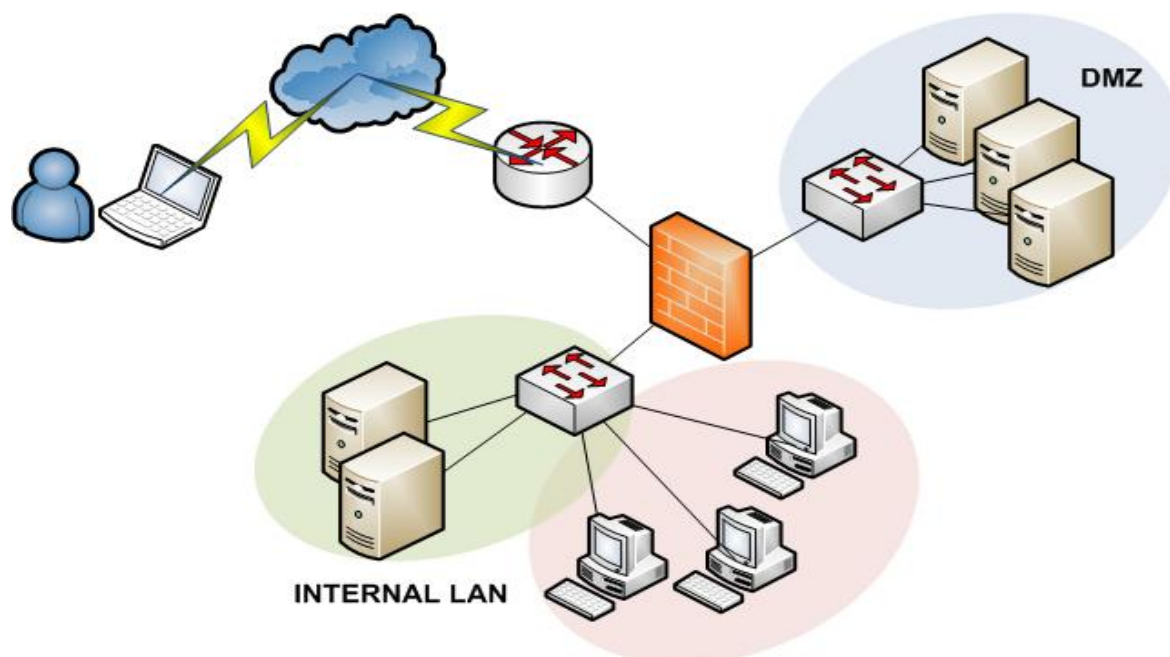
Figura 90: Topología de red objetivo
